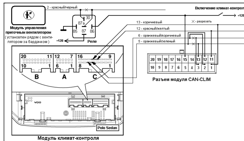
Рис. 6. Схема подключения модуля на а/м VW Polo Sedan.
