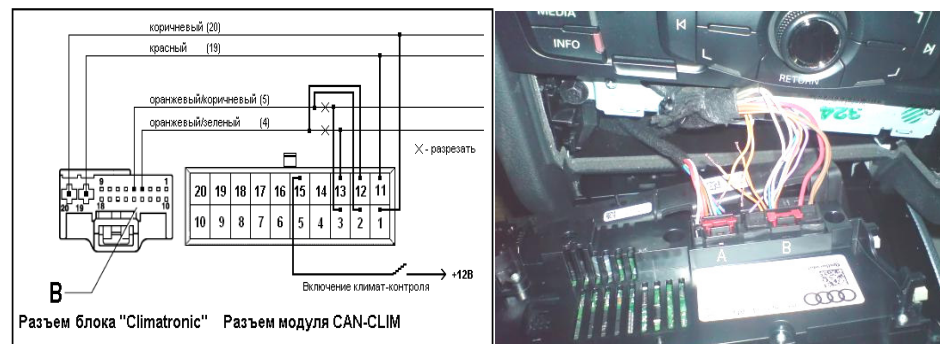
Рис. 4. Схема подключения модуля на а/м Audi A4, A5, Q5.
