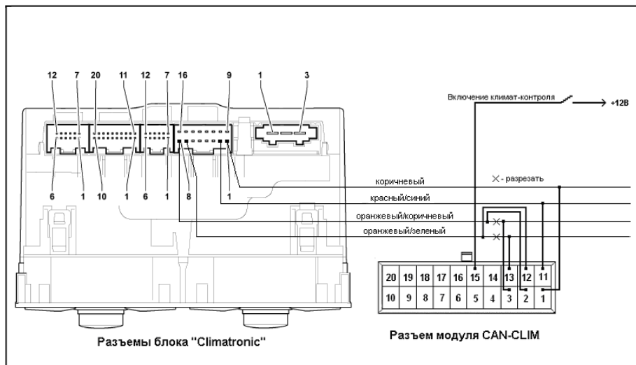
Рис. 3. Схема подключения модуля на а/м Audi Q7.
