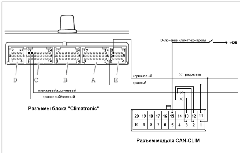
Рис. 2. Схема подключения модуля на а/м VW Touareg, T5.
