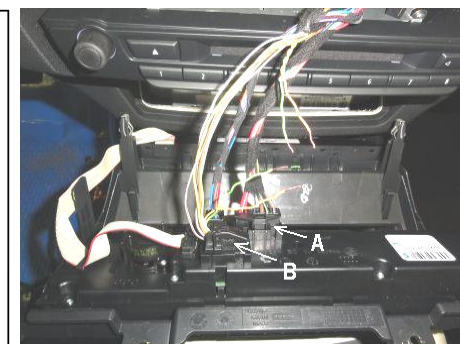
Рис. 5. Схема подключения модуля на а/м BMW.
