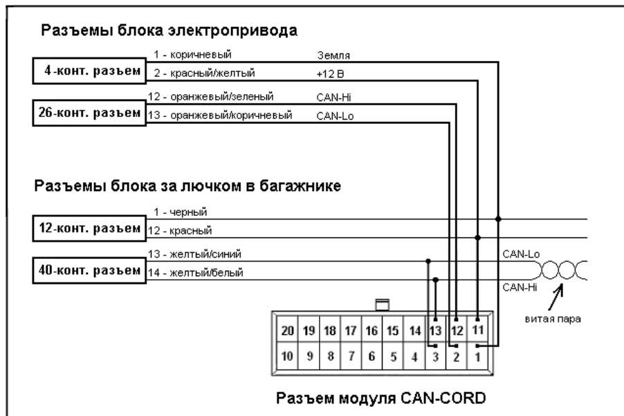
Рис. 2. Схема подключения модуля.
