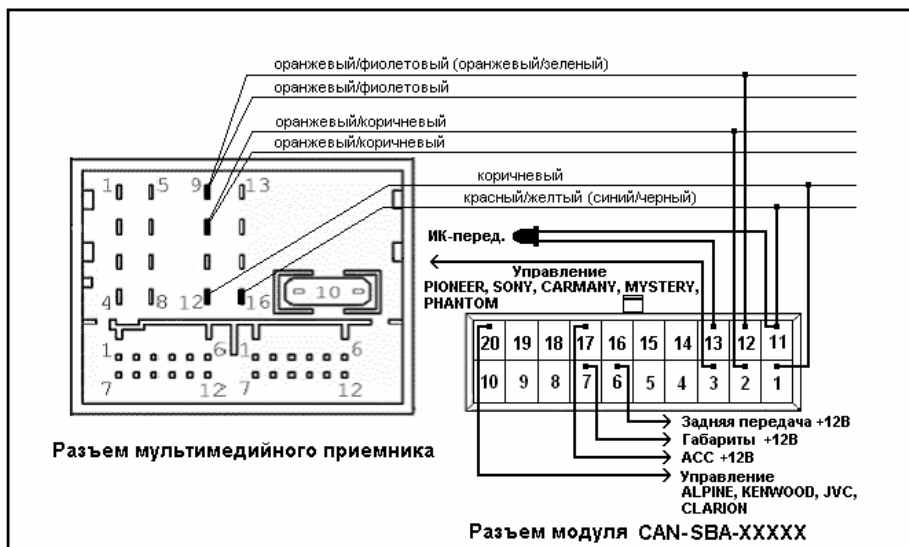
Рис. 1. Схема подключения модуля I
