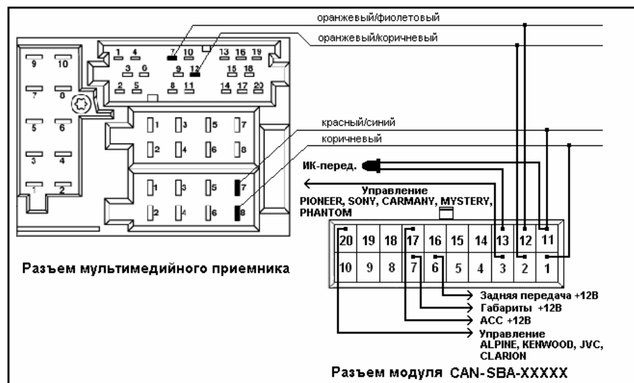
Рис. 2. Схема подключения модуля II
