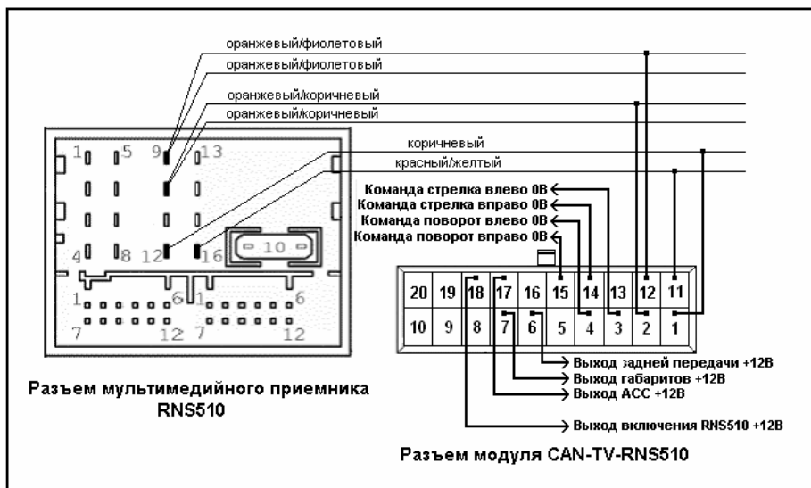
Рис. 1. Схема подключения модуля
